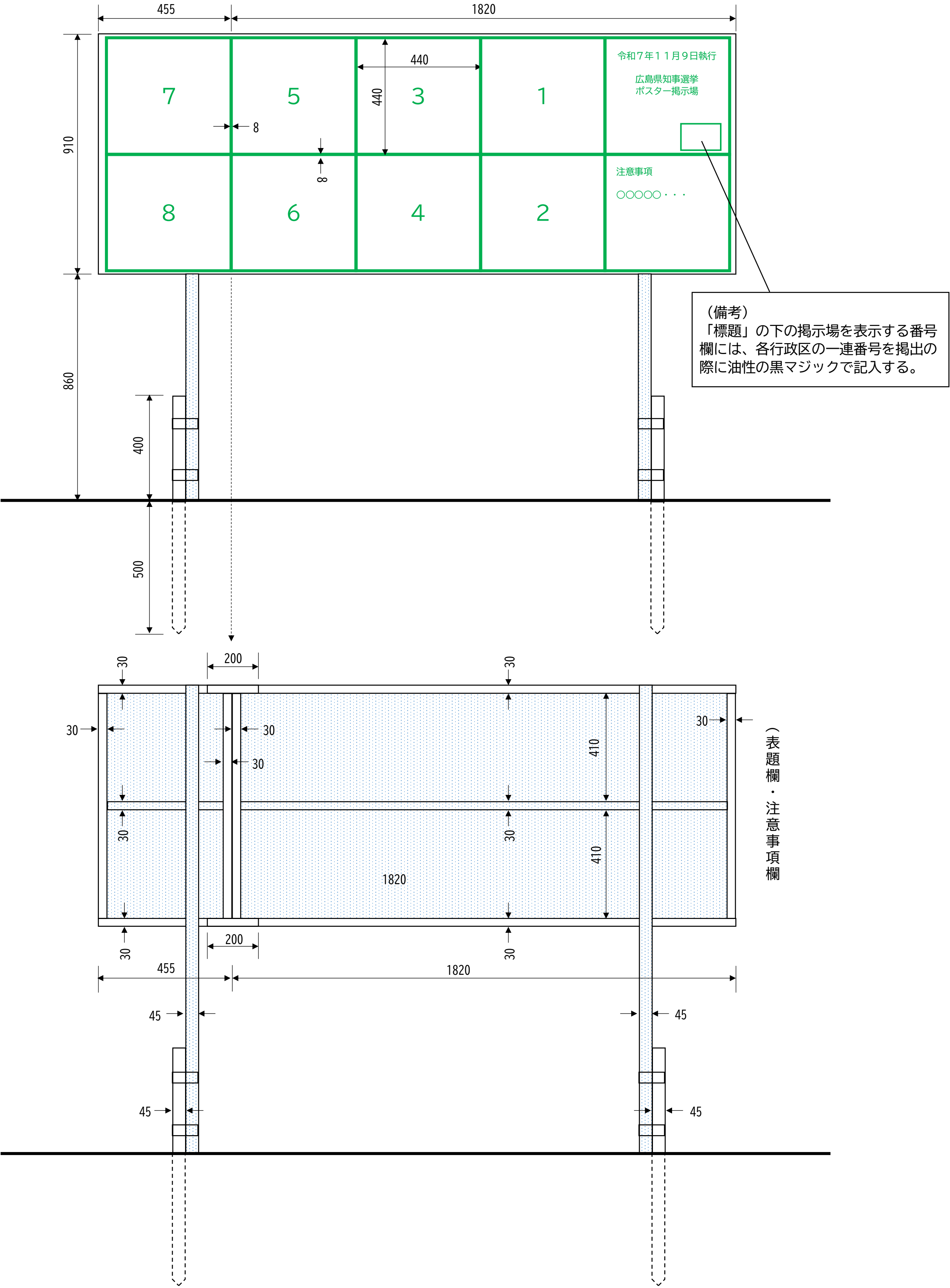
ポスター掲示場の設計図（8区画 正面図・裏面図）
