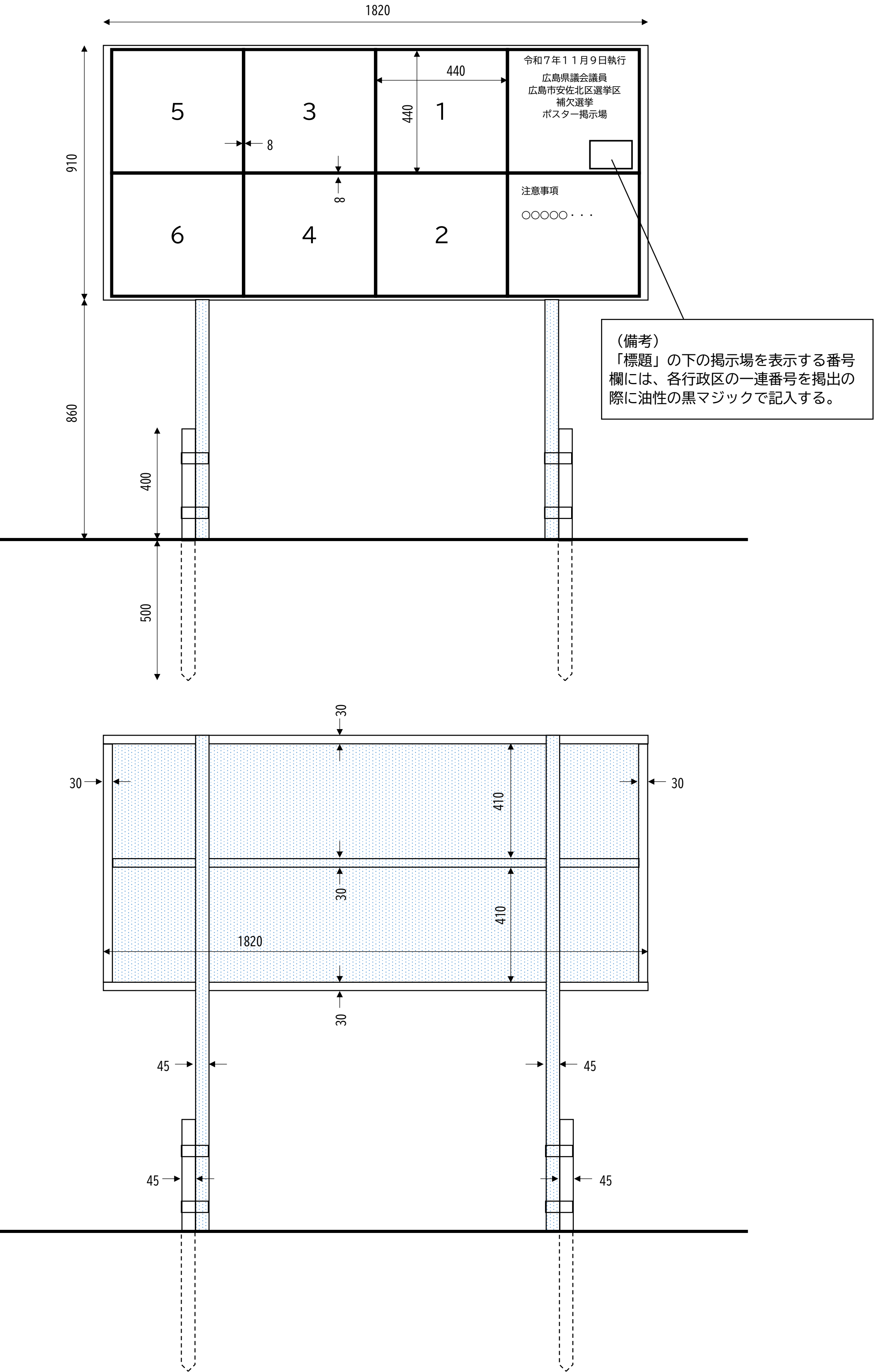
ポスター掲示場の設計図（6区画 正面図・裏面図）
