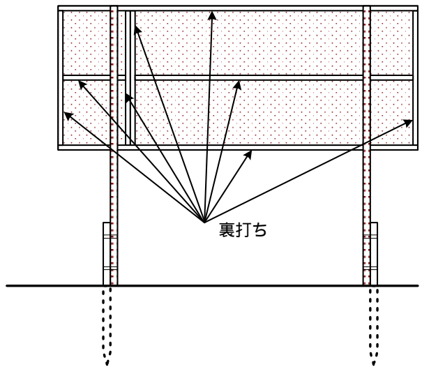
(裏面図)
