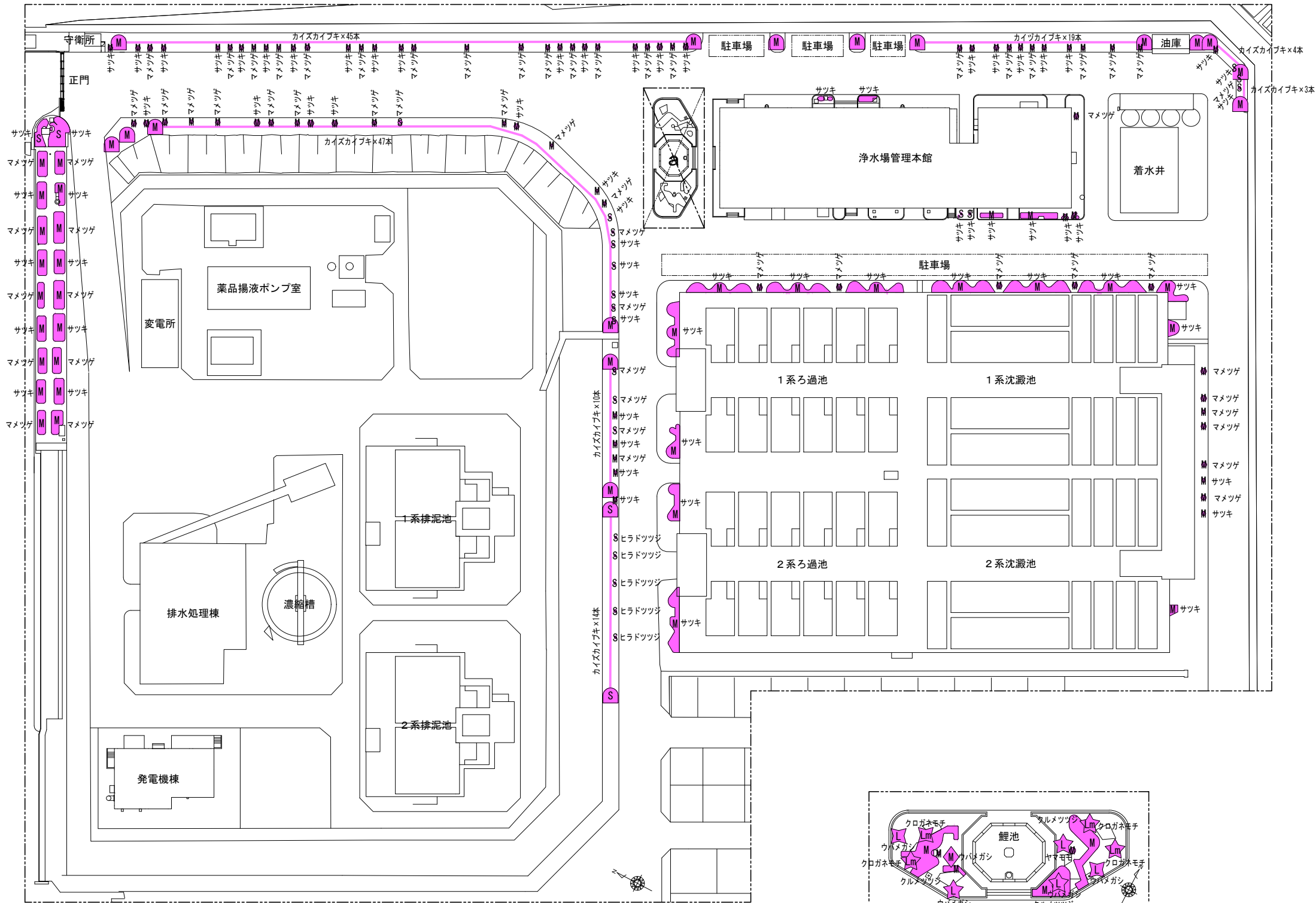
A部詳細 S=1/1,000
