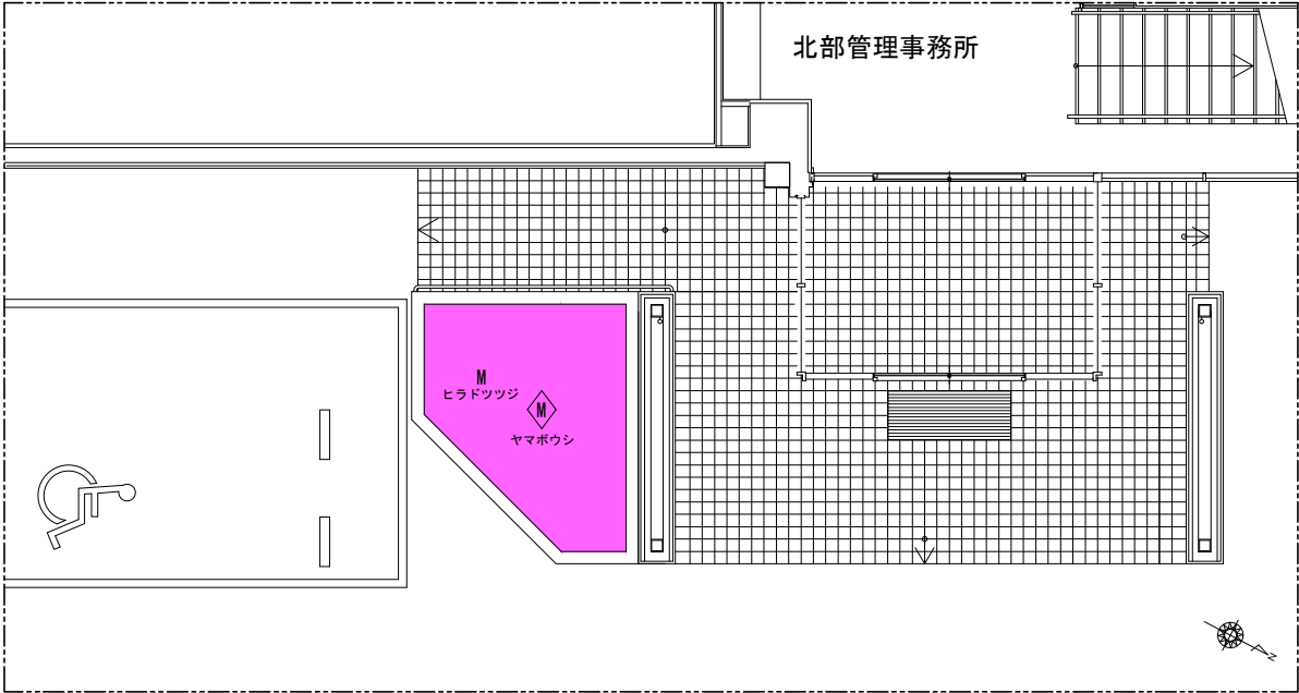
A部詳細 S=1/100
