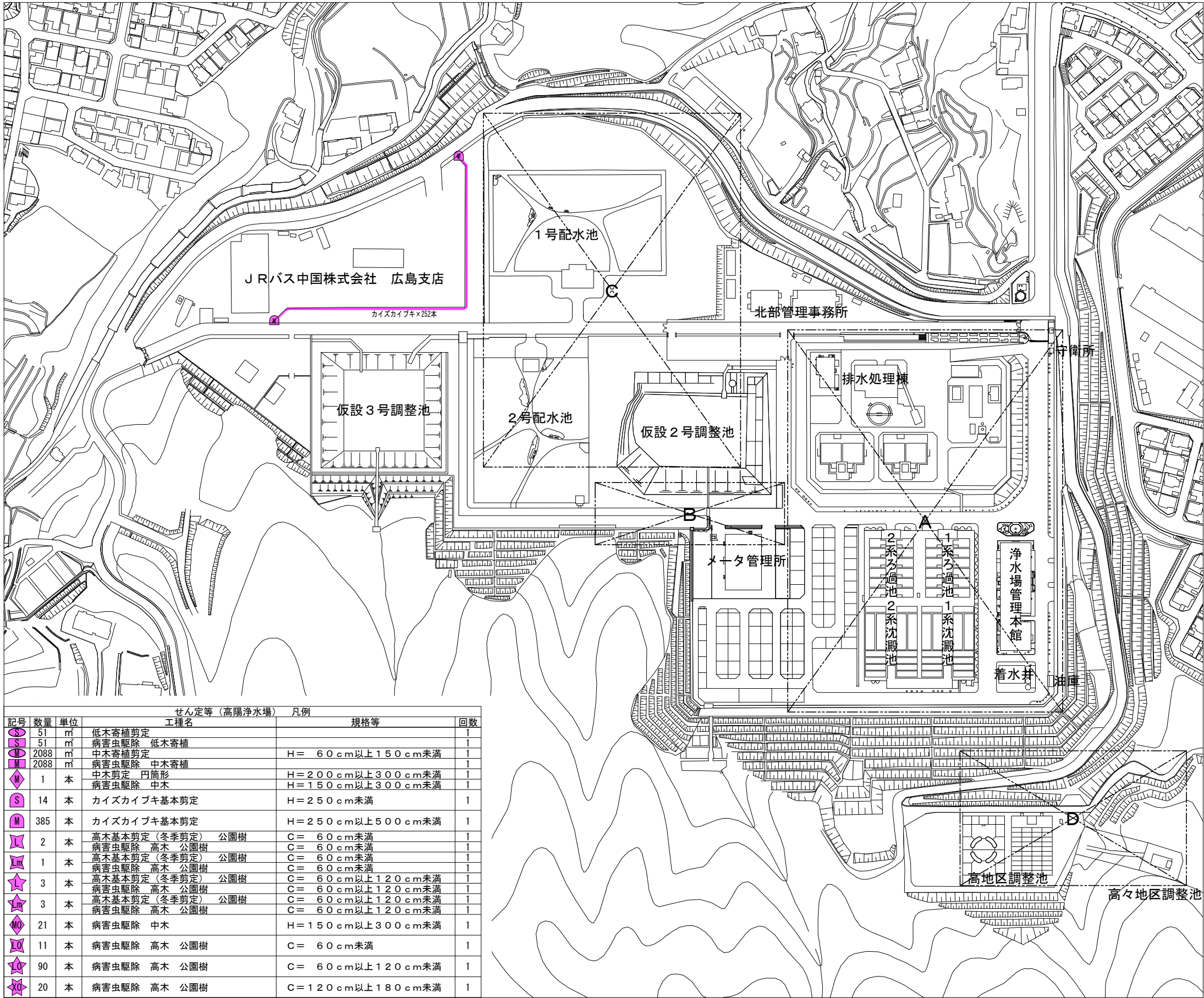
高陽浄水場平面図①
