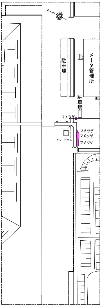
B部詳細 S=1/1,000
