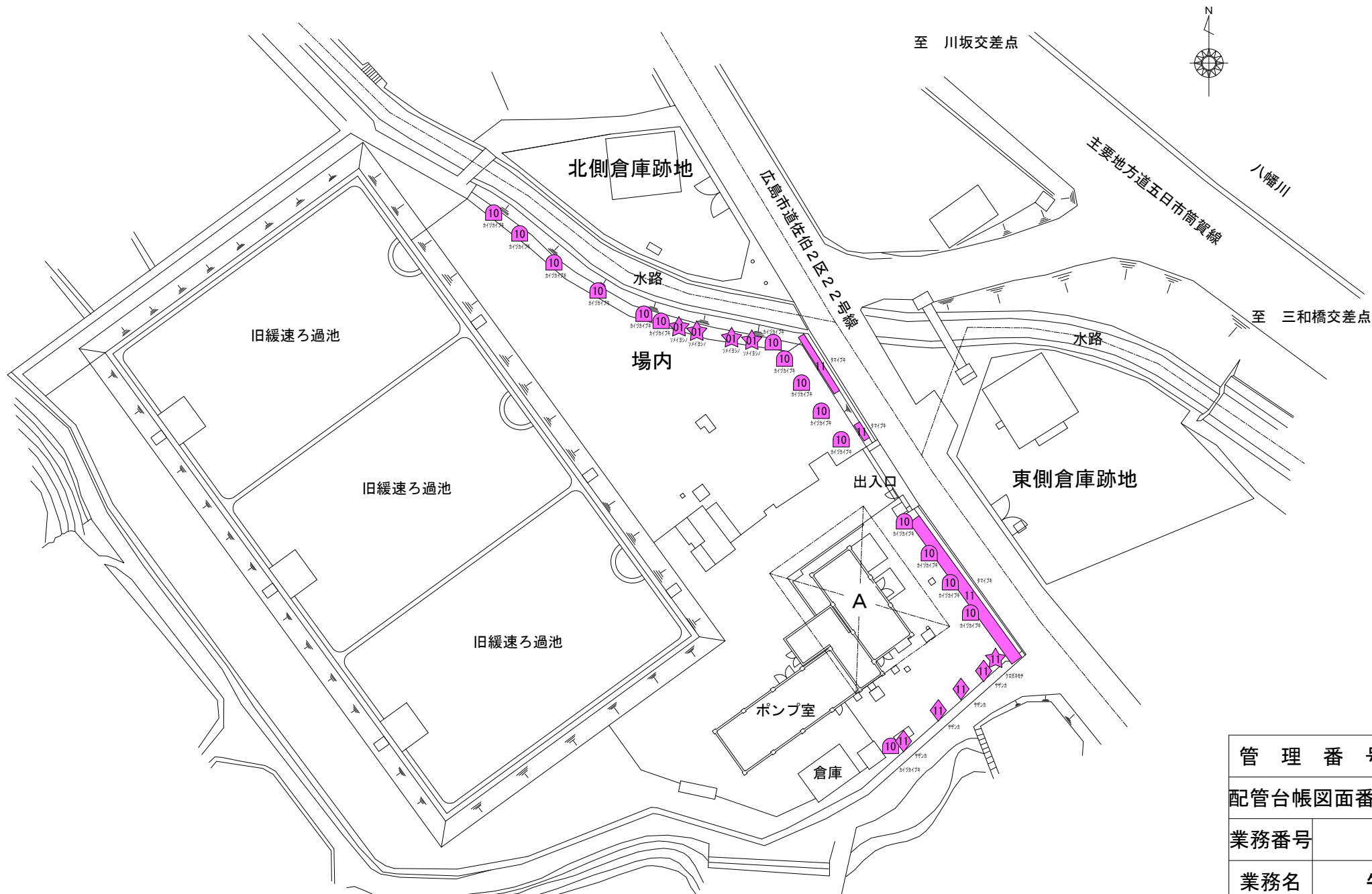
北原浄水場平面図 S=1/500
