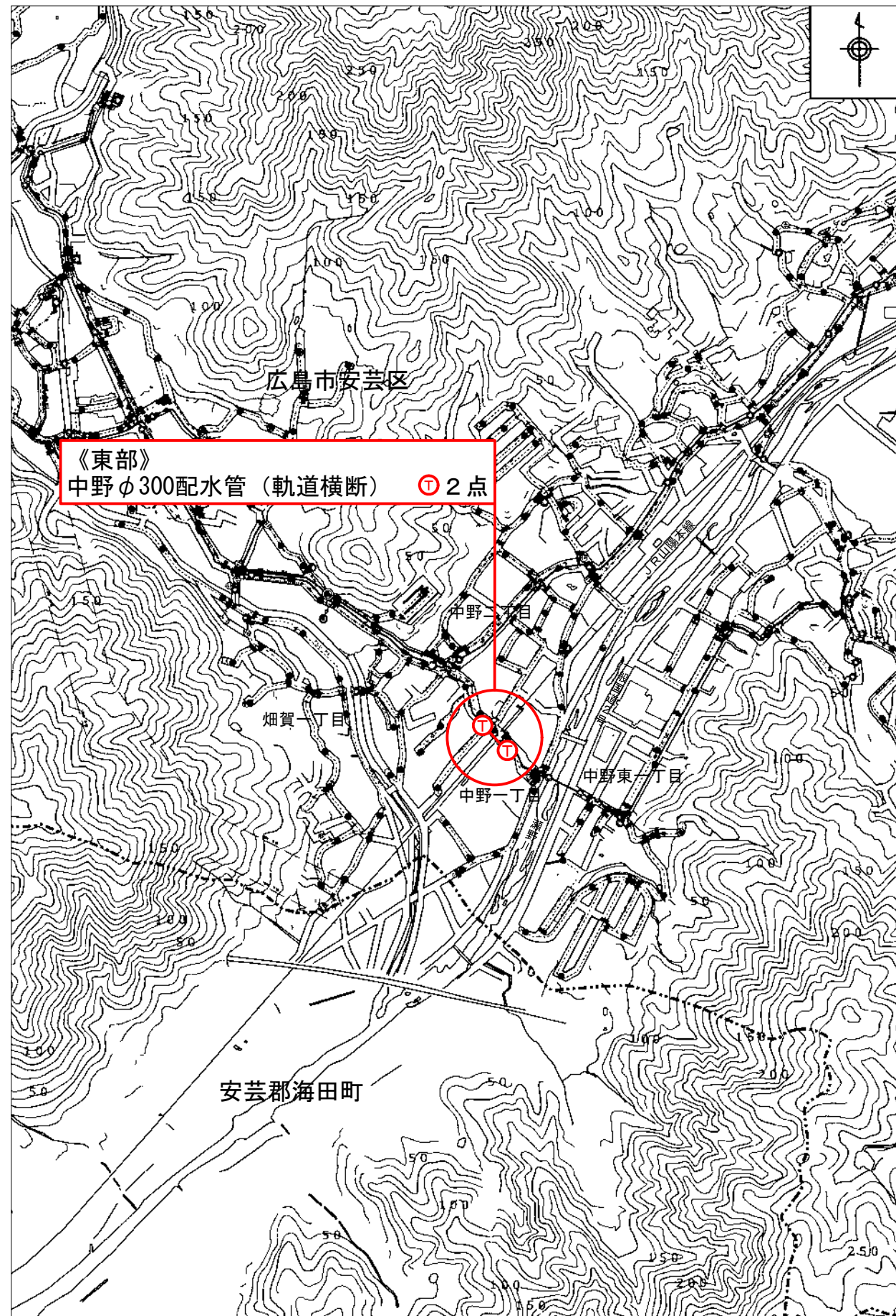
平面図(8) S=1/8,000
