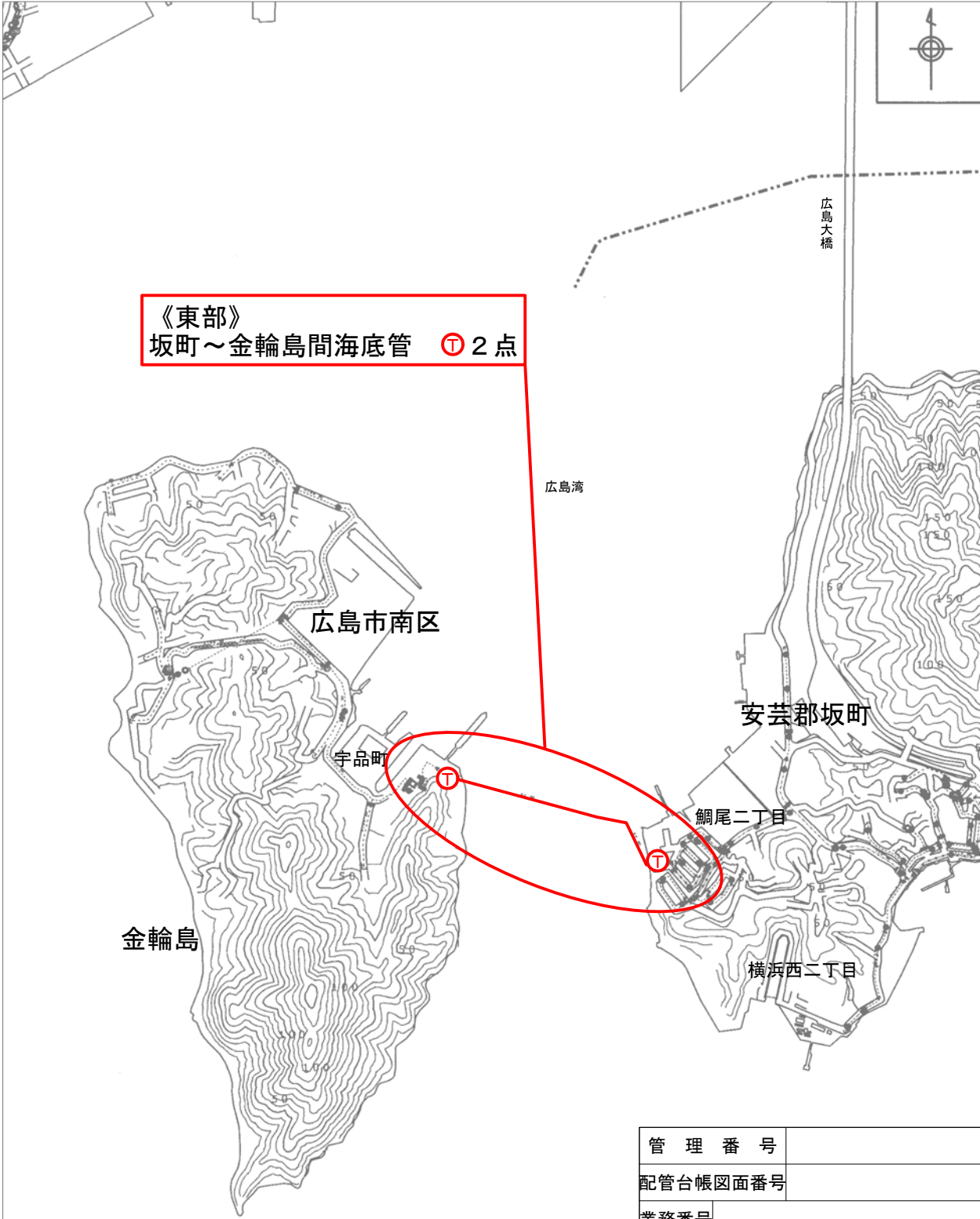
平面図(5) S=1/10,000
