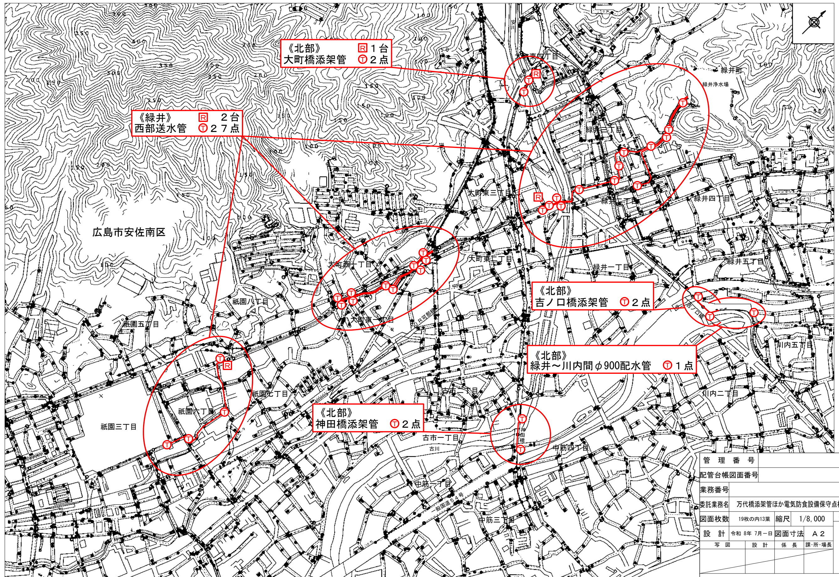
平面図(14) S=1/8,000
