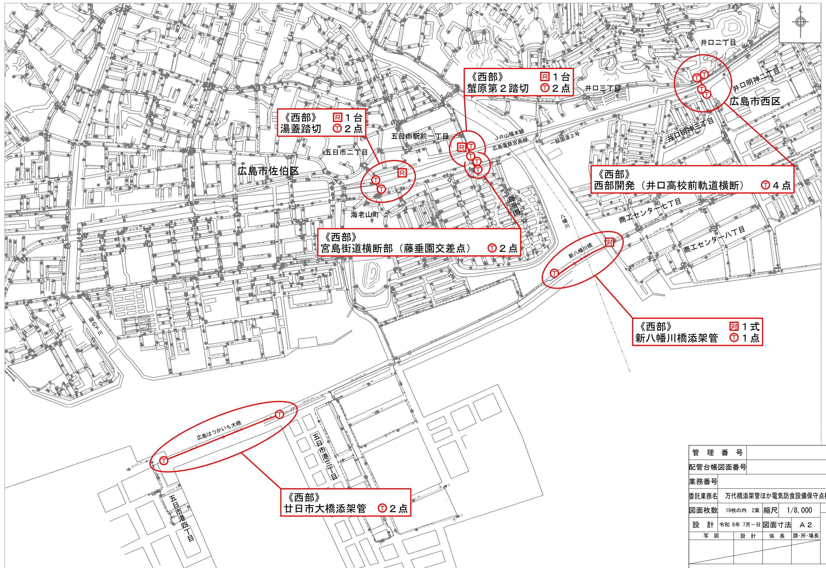
平面図(1) S=1/8,000
