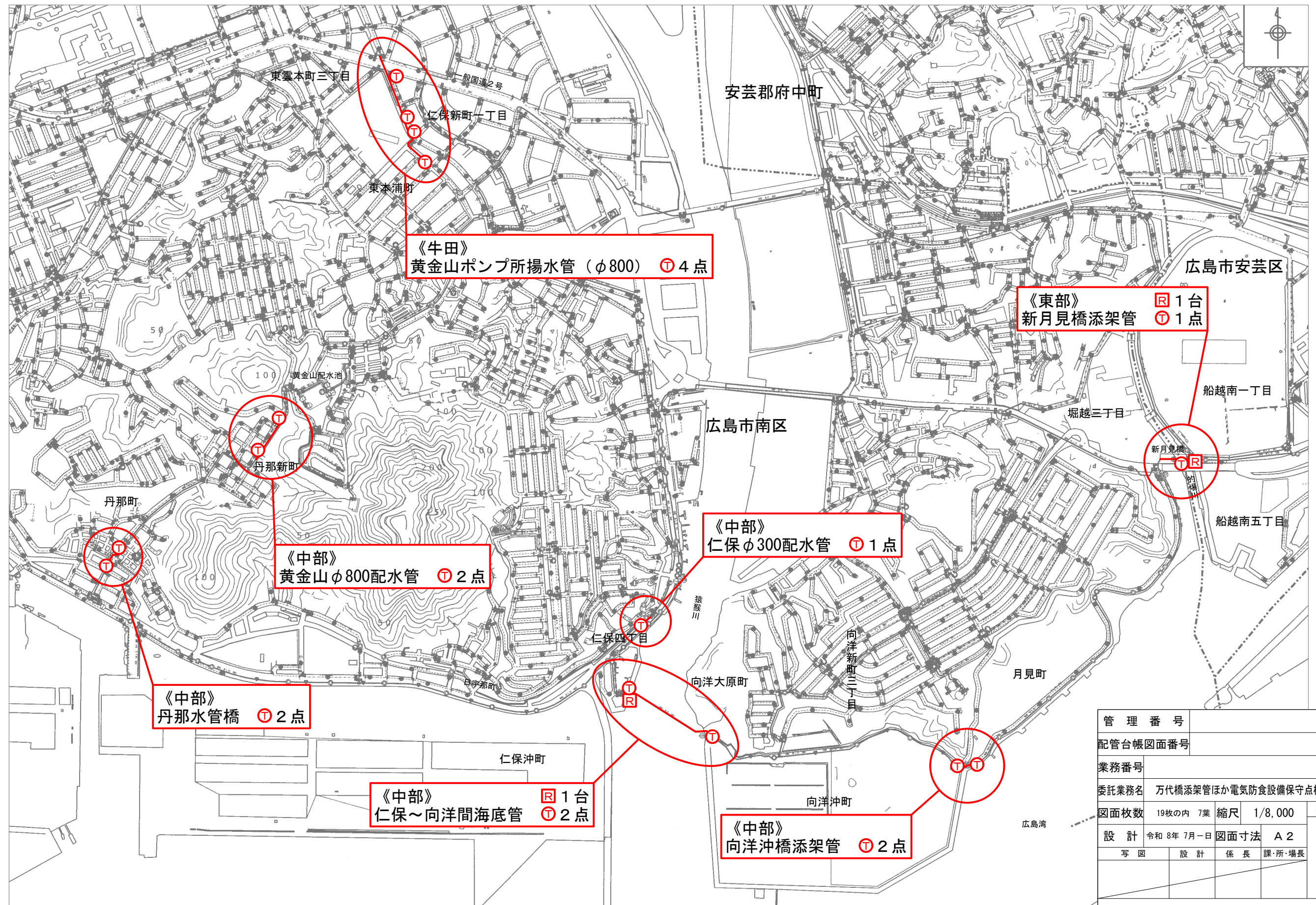
平面図(7) S=1/8,000
