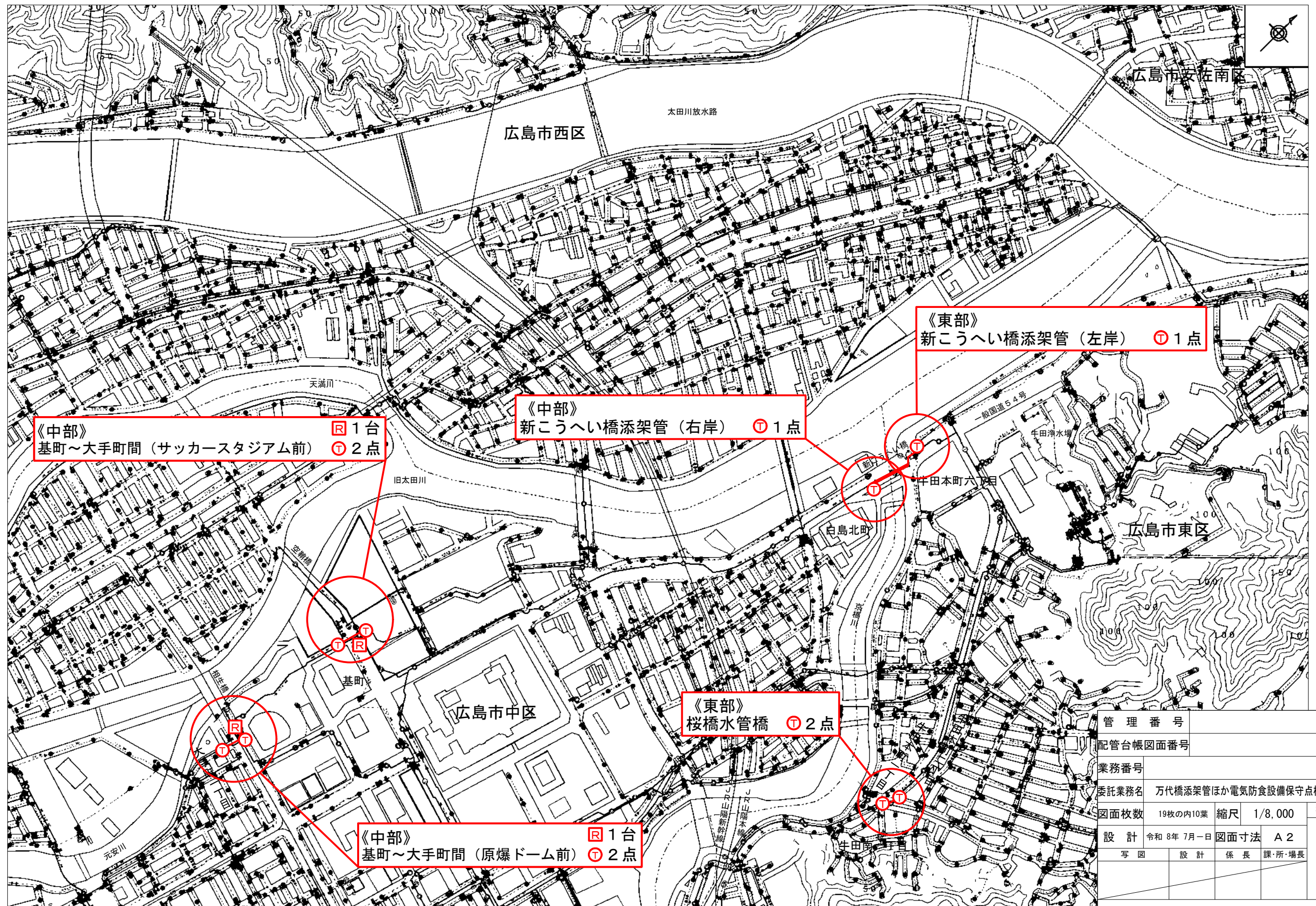
平面図(11) S=1/8,000
