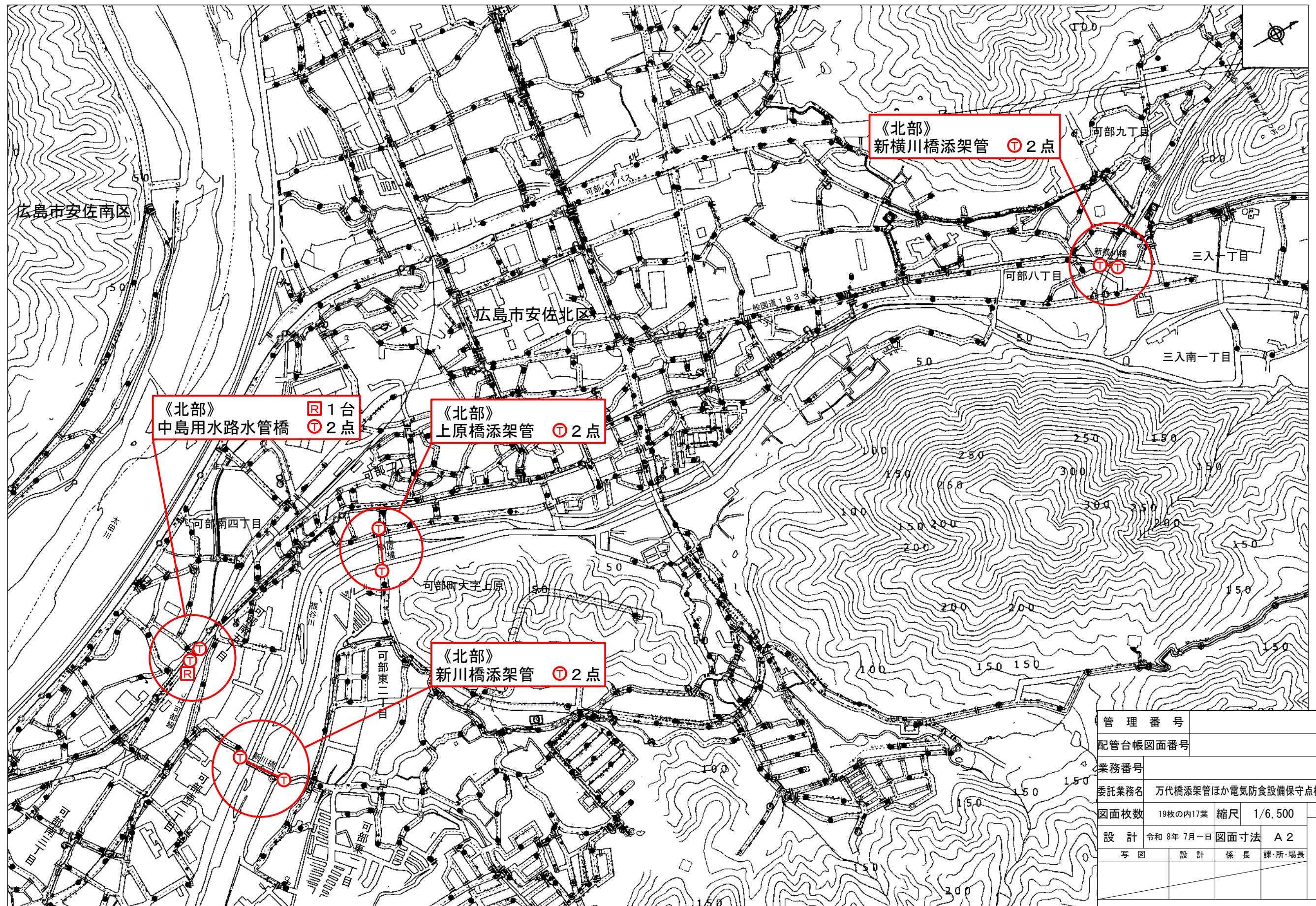
平面図(18) S=1/6,500
