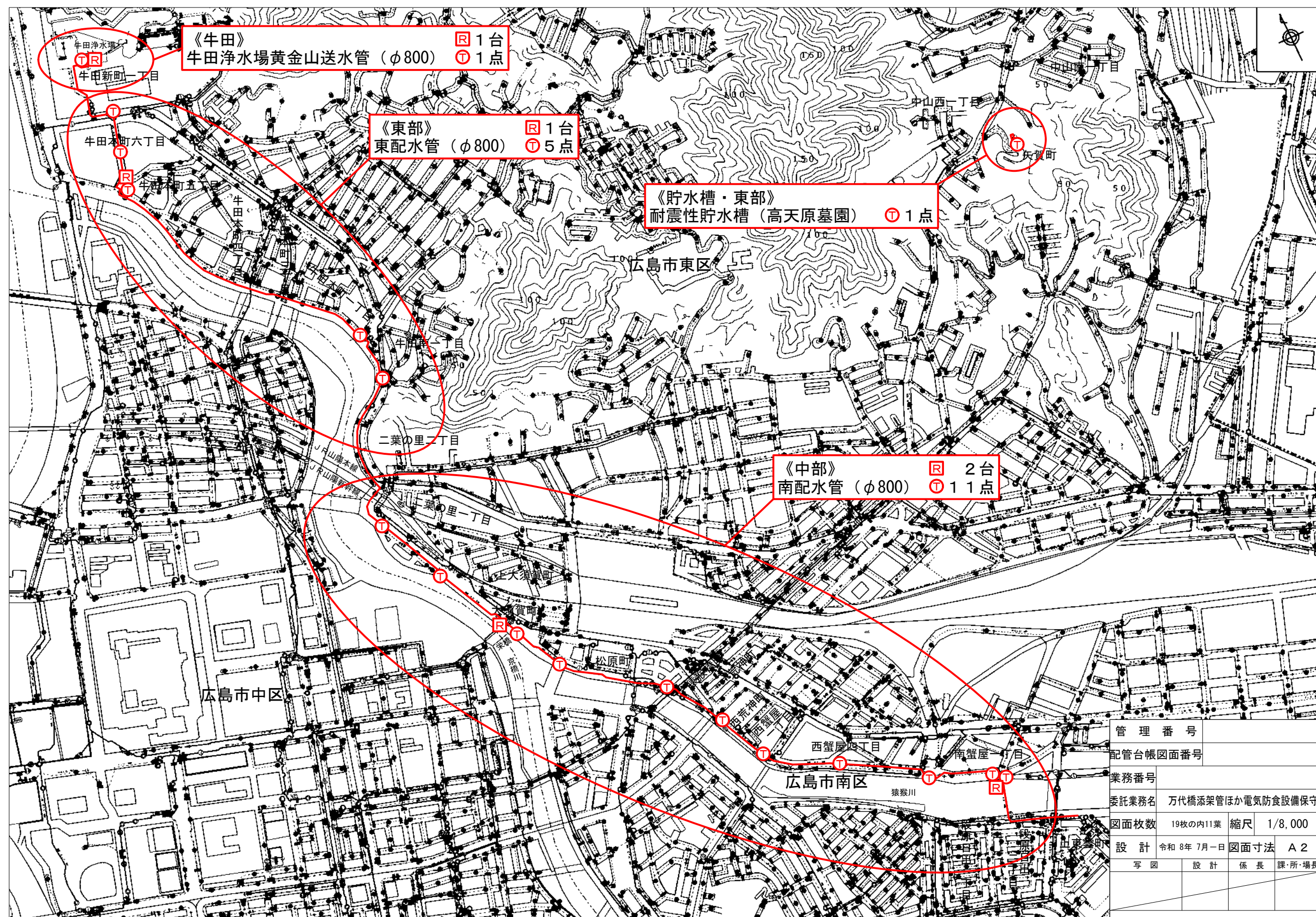
平面図 (12) S=1/8, 000
