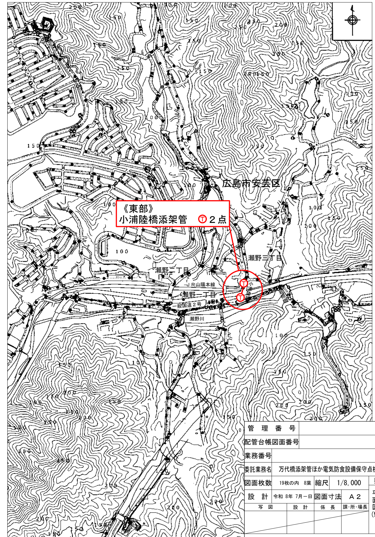
平面図(9) S=1/8,000
