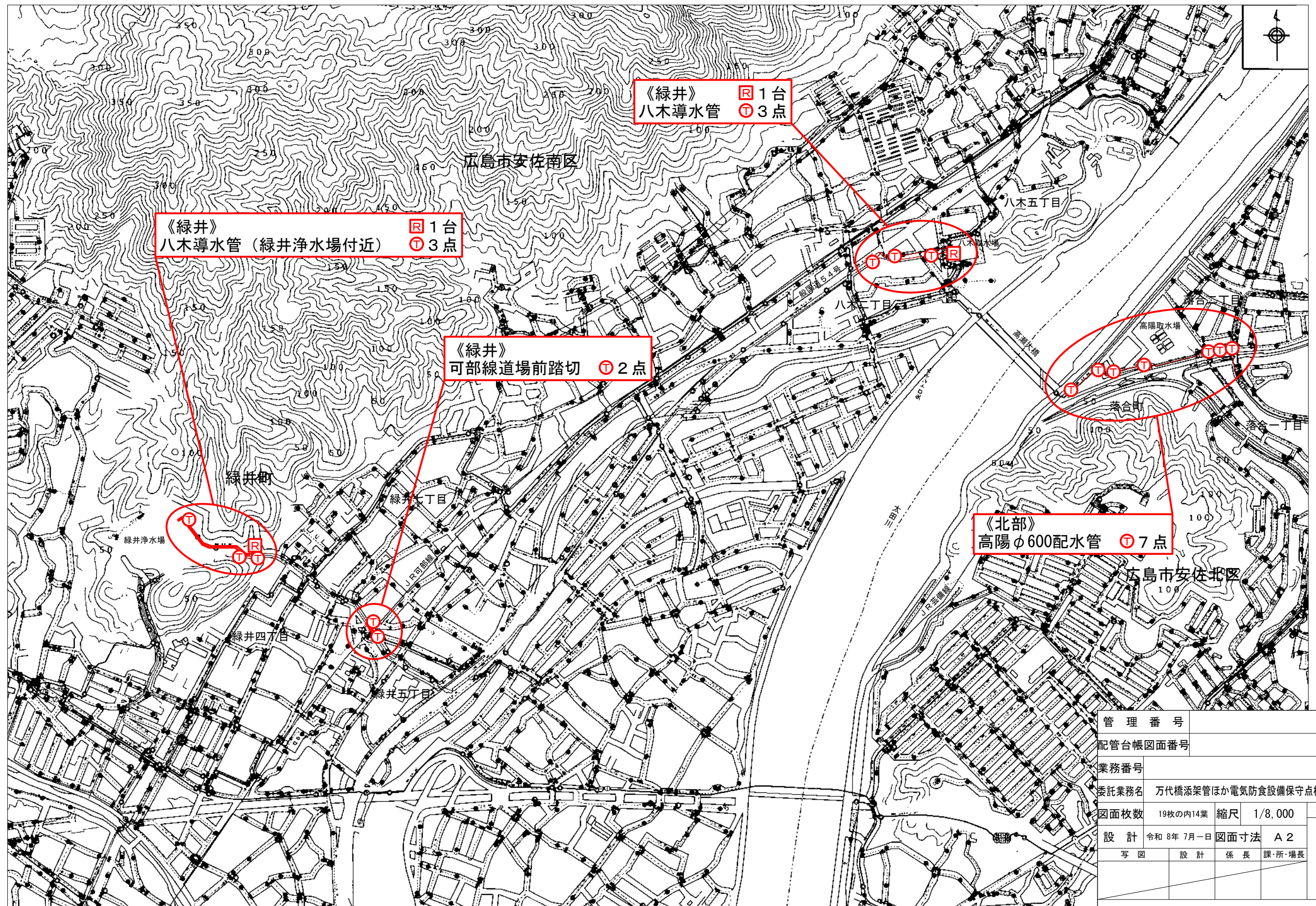
平面図(15) S=1/8,000
