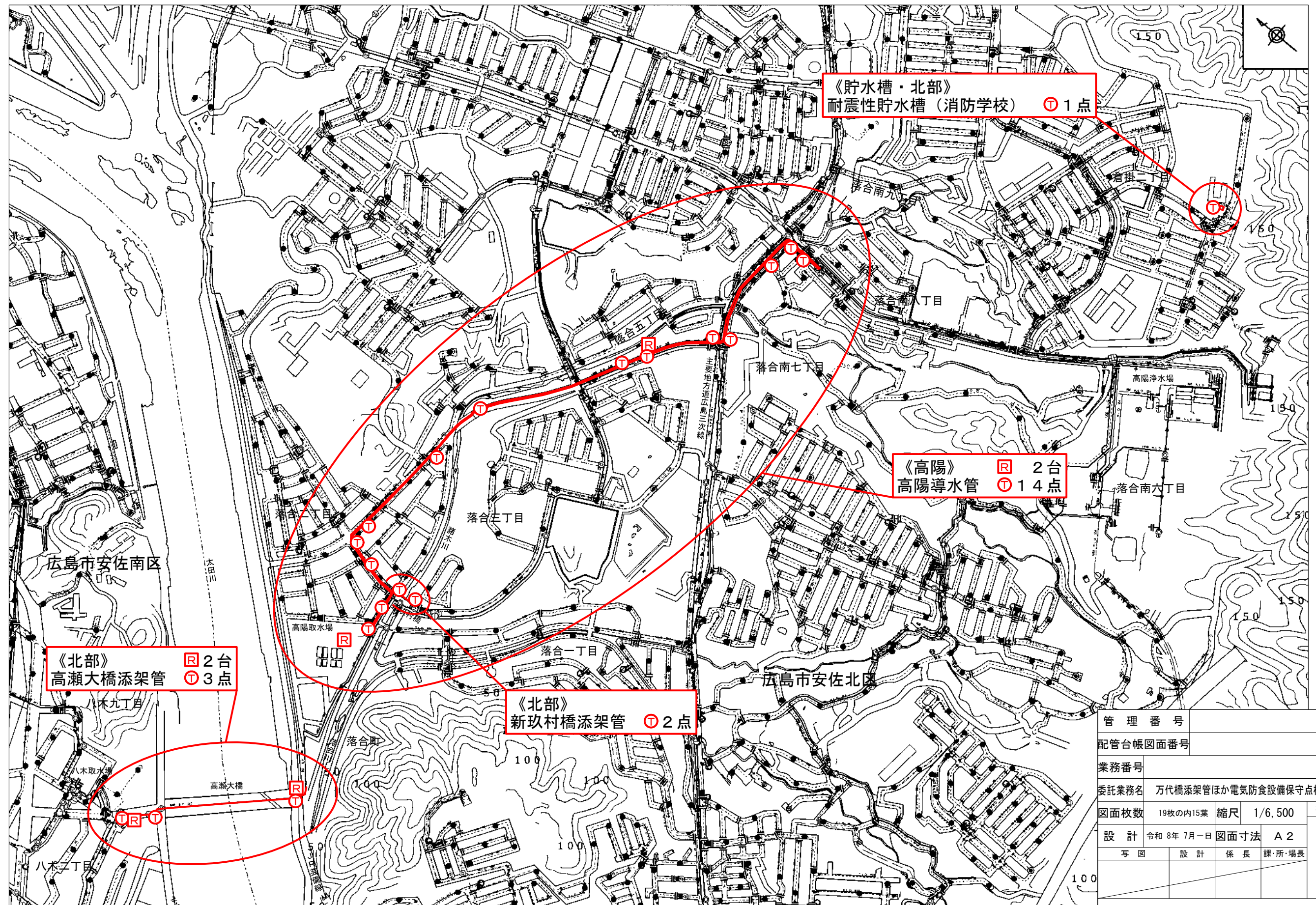
平面図(16) S=1/6,500
