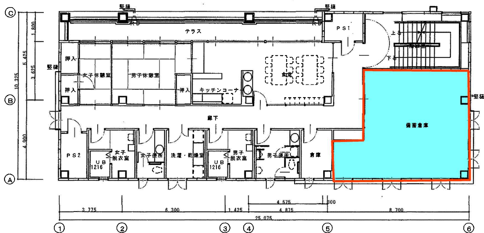
3階平面図
