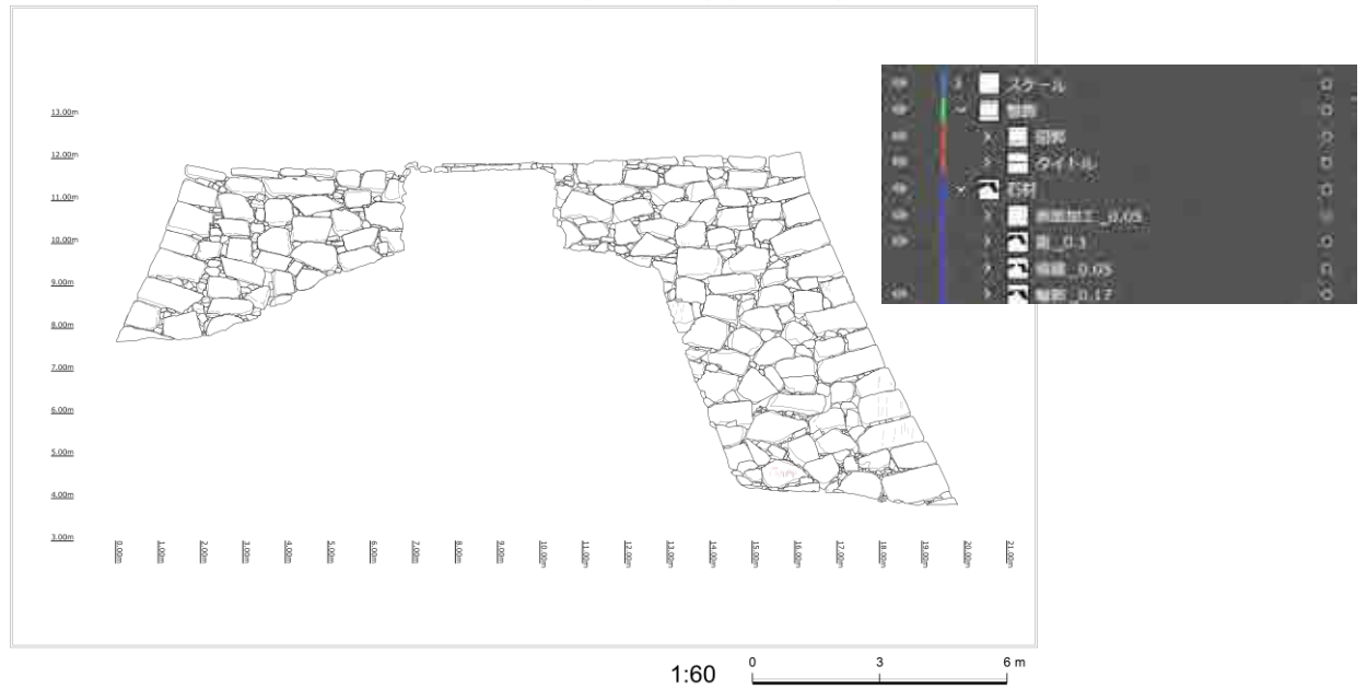
広島城小天守台石垣現況調査業務 石垣立面図 石垣⑩(H51・H52) (S= 1/60 )
