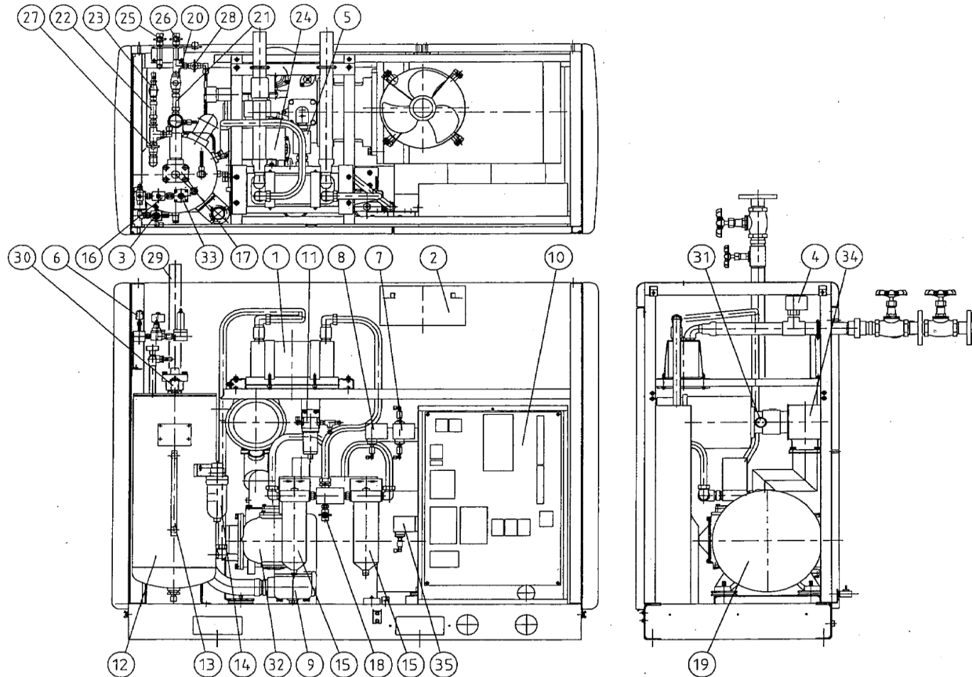
計装用空気圧縮機組立図
